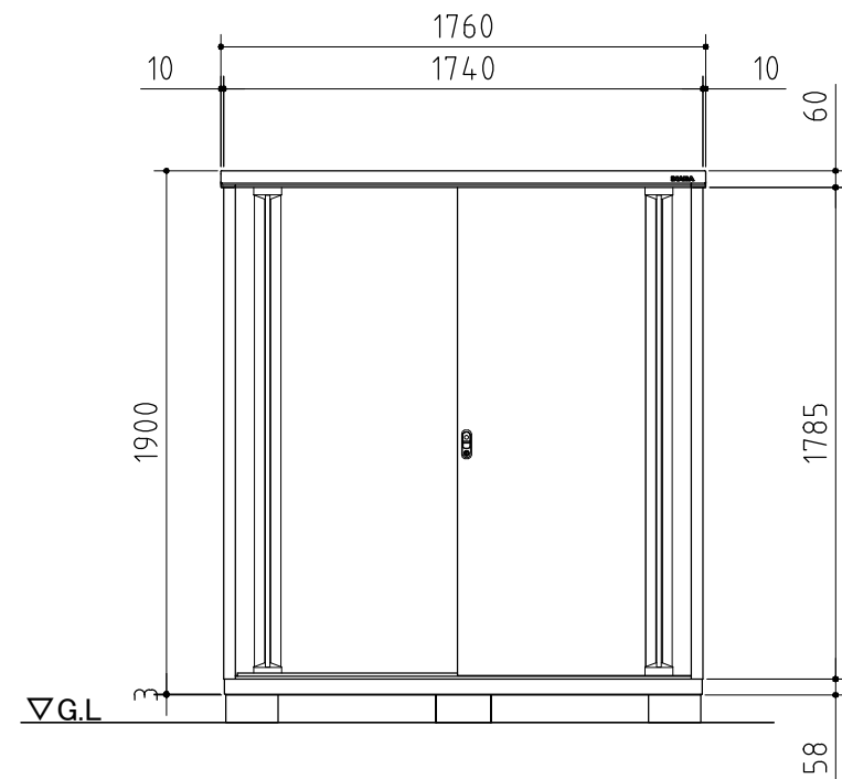
正面図
