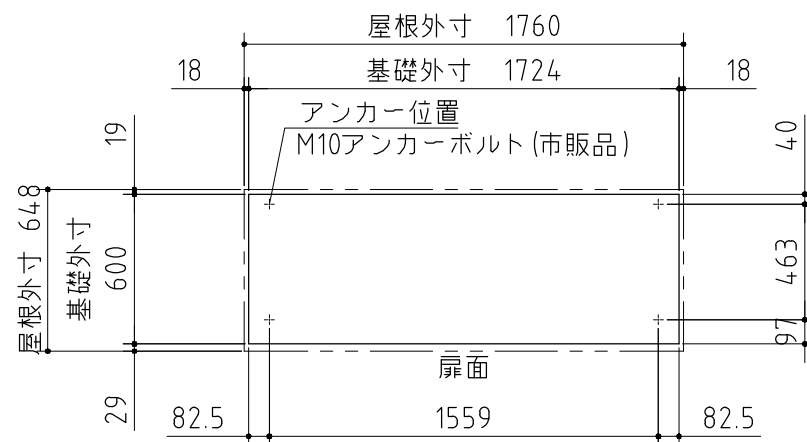
ベタ基礎図
